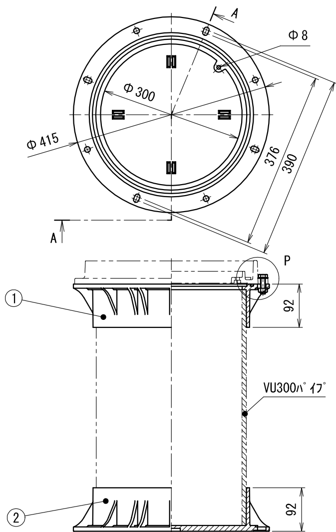
A-A断面図
